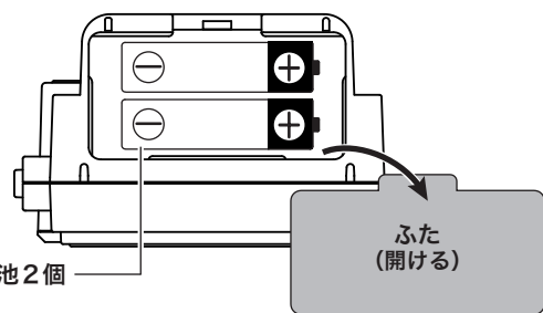
【底面】
