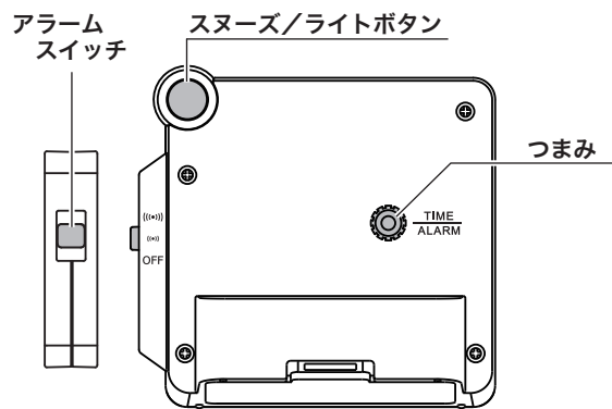
【裏面】
